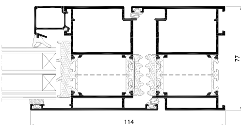
przekrój drzwi MB-86 SI+
